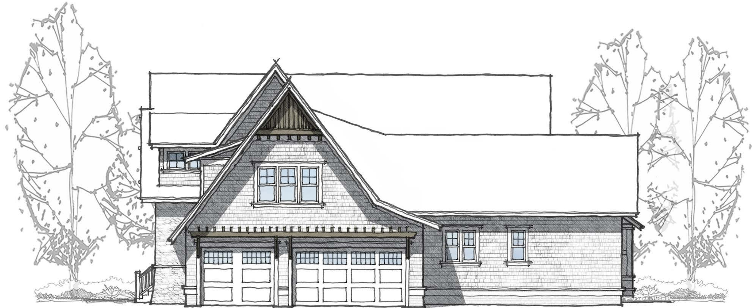
RIGHT ELEVATION
